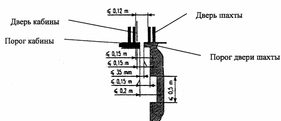
Рис.3 Расстояния между элементами кабины и шахты
