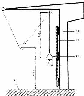
Рис. 3. Высота падения на испытательном стенде
