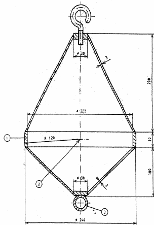
Рис. 1. Маятник для жесткого удара
