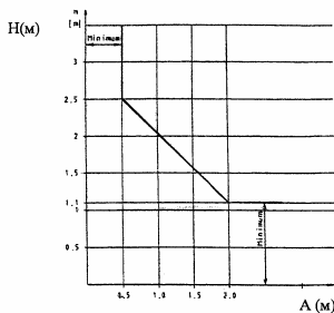
Рис.2 Высота ограждения шахты в зависимости от расстояния до движущихся элементов лифта
