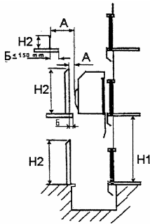
Рис.1 Расстояние до движущихся элементов лифта
