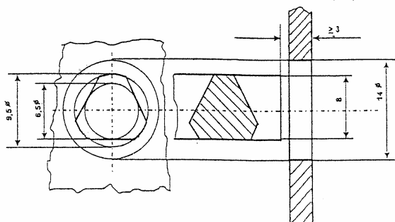
"Размеры ключевины устройства отпирания замка (мм)"
