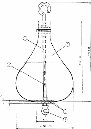
Рис. 2. Маятник для нежесткого удара
