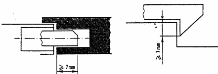
Рис. 5. Запирающее устройство автоматического замка двери шахты
