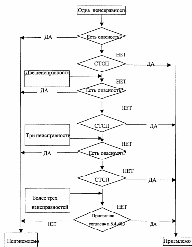
Рис. 6 Блок-схема оценки электрических схем безопасности.
