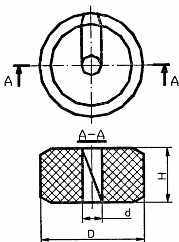
Рис. П6.2. Кольцо для уплотнения кабелей
